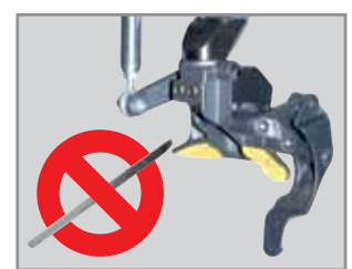
Bec de montage / démontage sans levier (breveté) Mounting / demounting without lever (patented)
